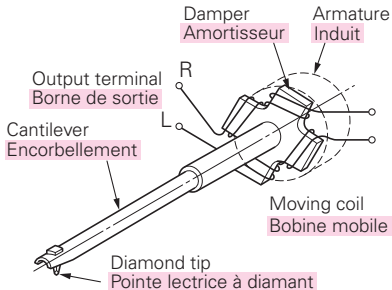
Fig. 4 Construction Sketch Fig. 4 Schéma de construction
